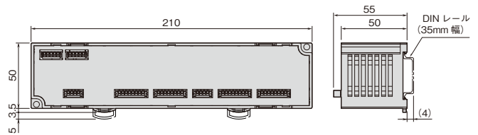
外形寸法図 (単位: mm) 機種により外觀が若干異なります。
