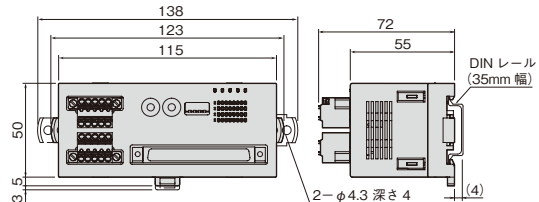
外形寸法図 (単位: mm) 機種により外觀が若干異なります。
