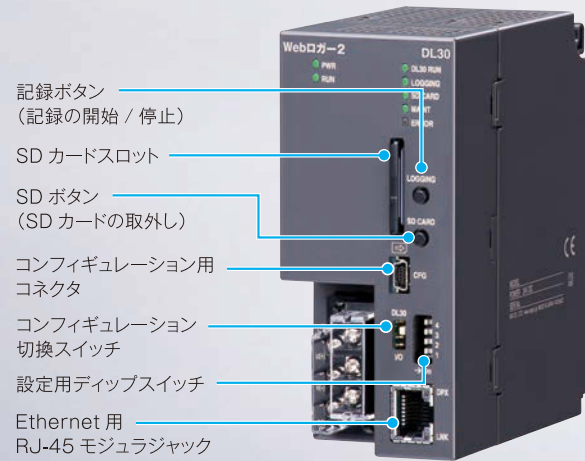
Web ロガー 2 本体
